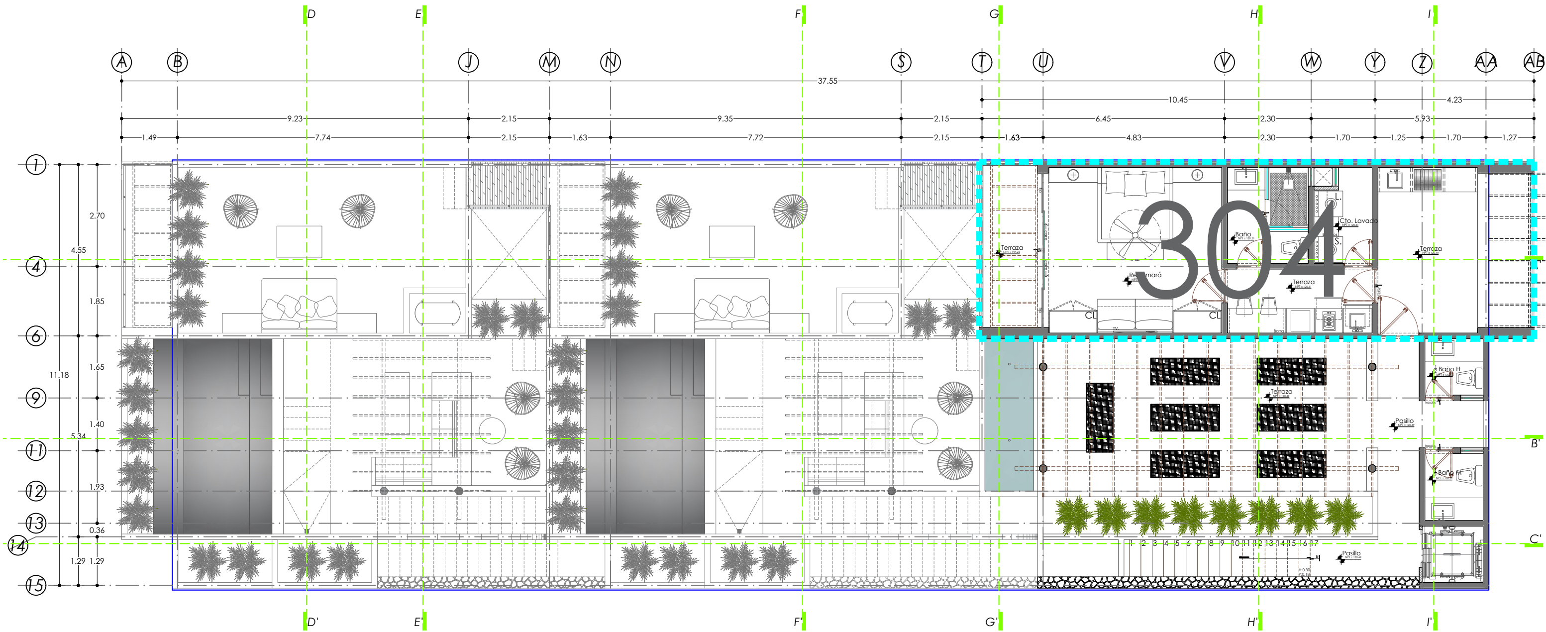
PLANTA DE AZOTEA ROOF TOP ESCALA (Scale): 1:100
